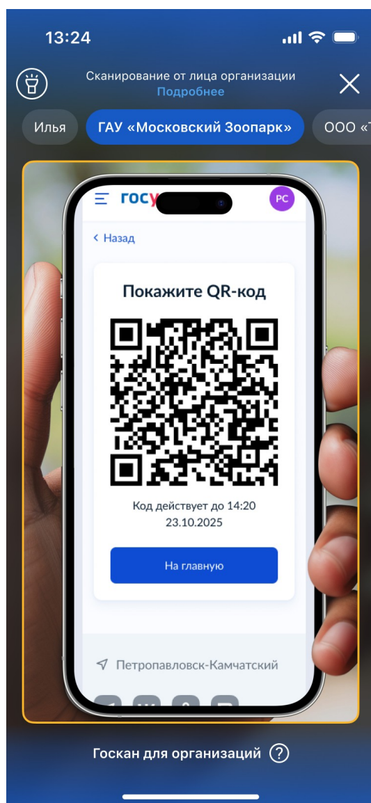
Рисунок 5. Сканирование QR-кода
