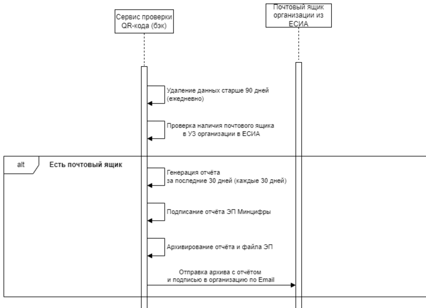
Рисунок 15. Схема информационных потоков при отправке отчёта о сканировании в организации.
